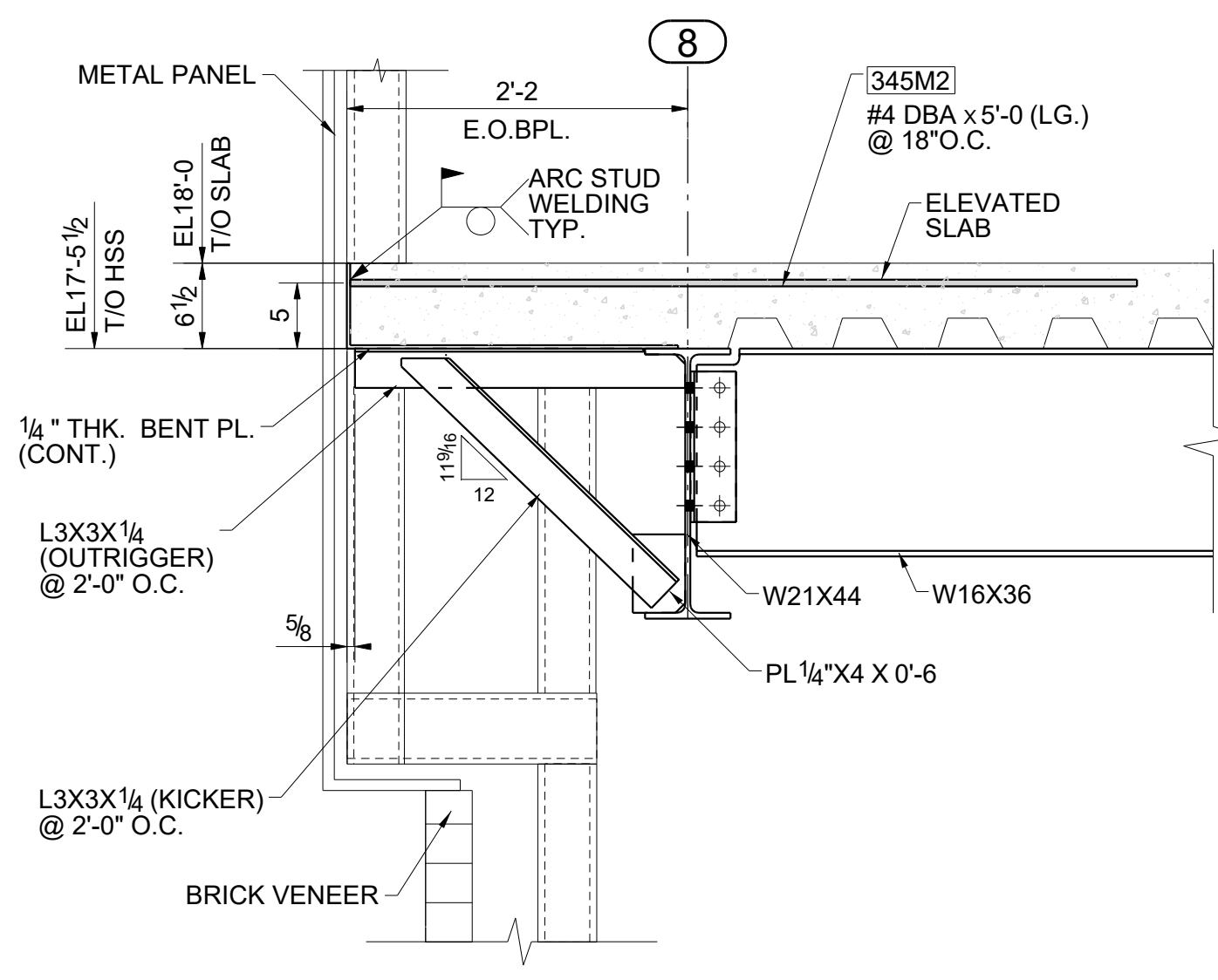
SECTION 12 - 12 E102 (REFER:SECTION 4/S5.006)
