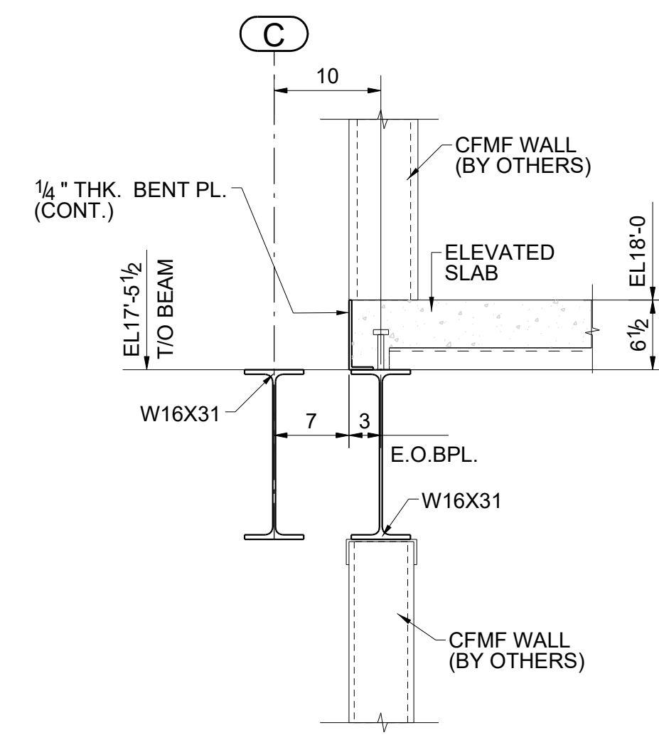
SECTION 13 - 13 E102 (REFER:SECTION 5/S5.006)
