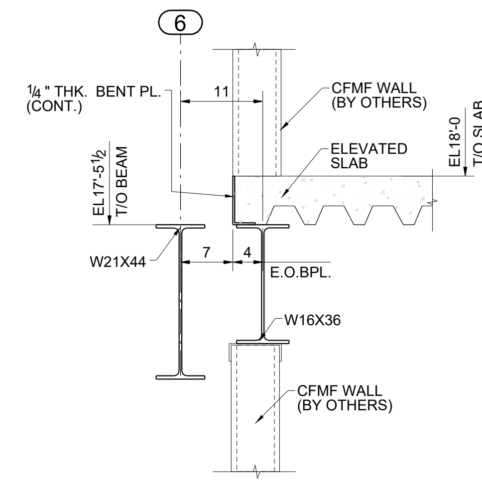
SECTION 14 - 14 E102 (REFER:SECTION 6/S5.006)
