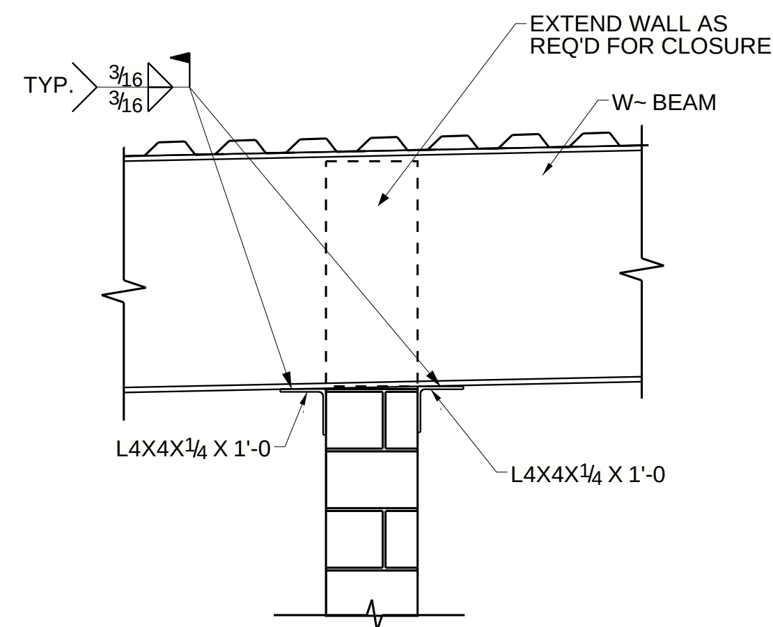
SECTION 32 - 32 E104
