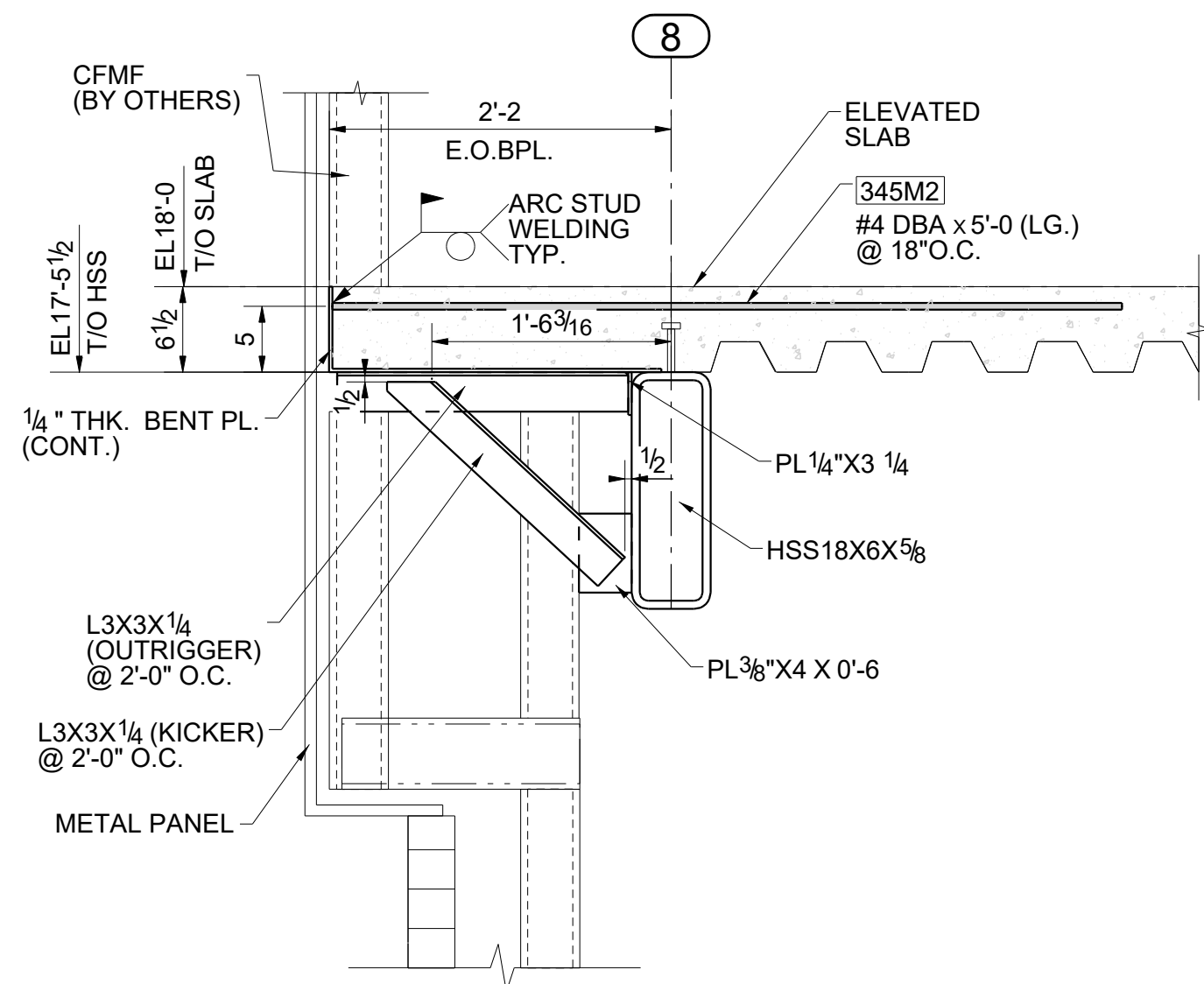
SECTION 11 - 11 E102 (REFER:SECTION 2/S5.006)
