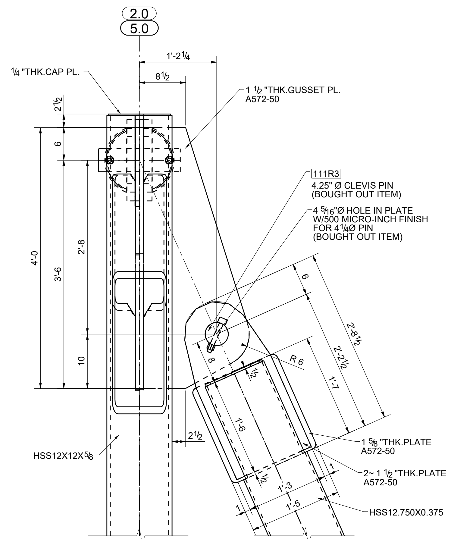
SECTION 56A - 56A
