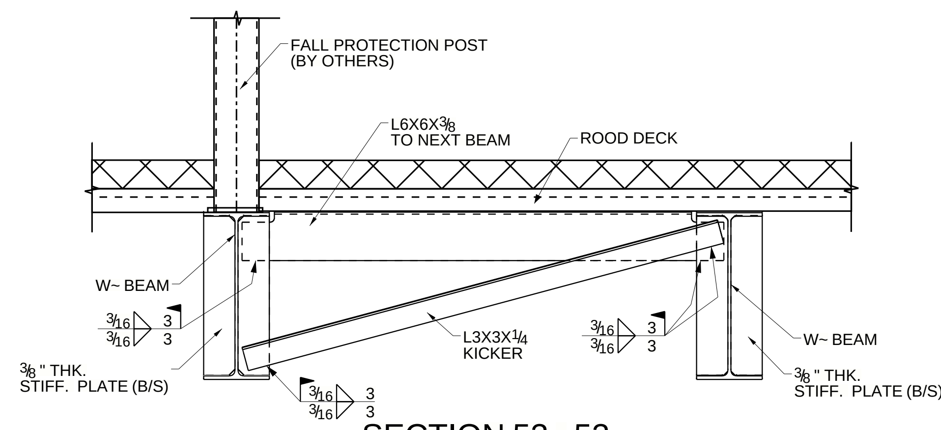
SECTION 53 - 53 E102
