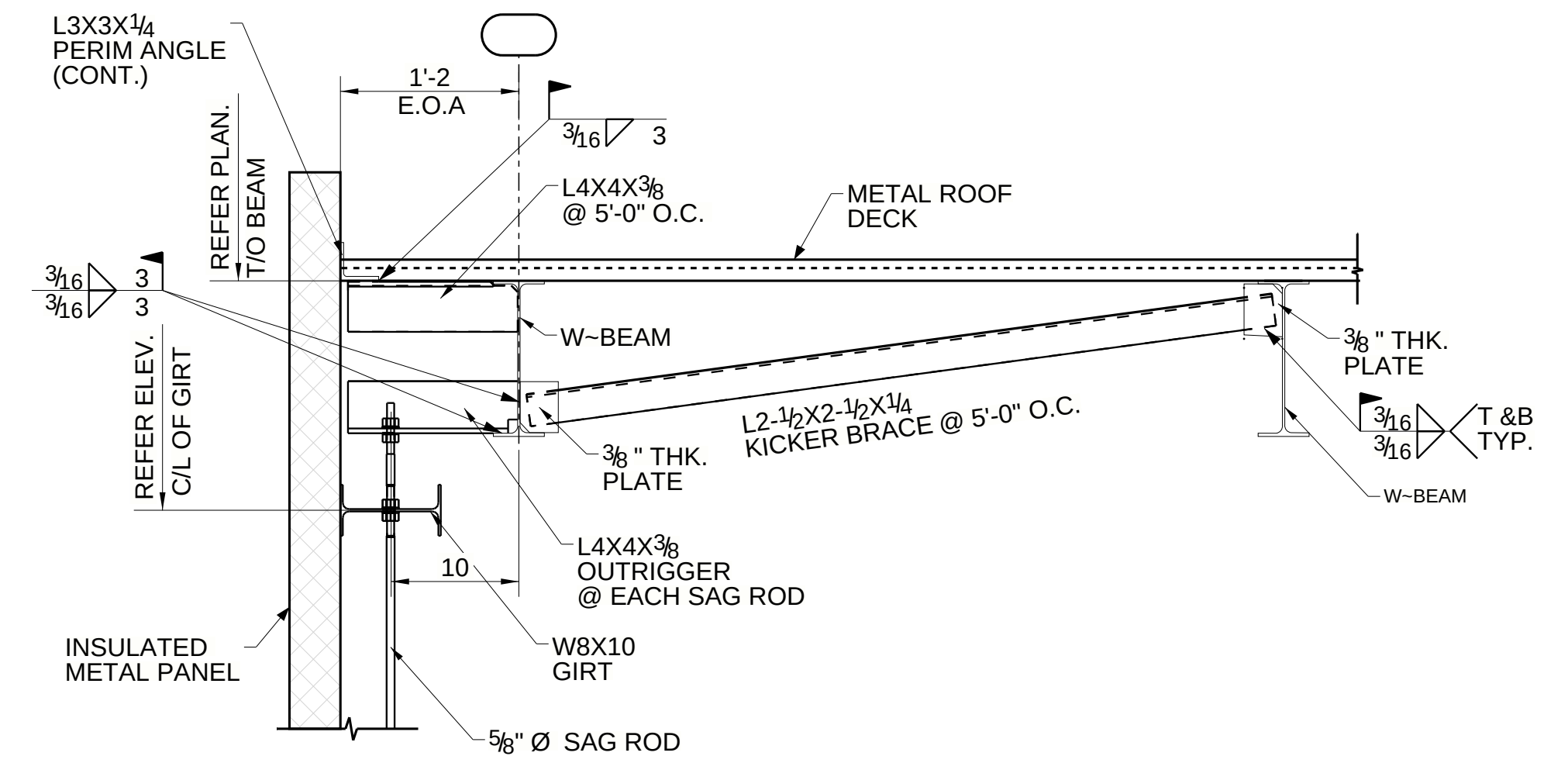
SECTION 30 - 30 E103
