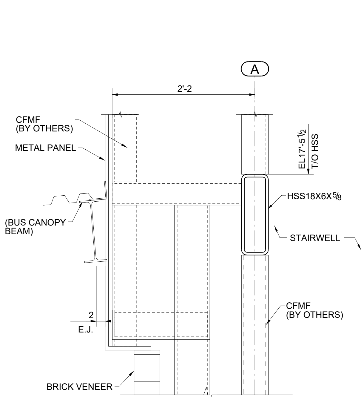
SECTION 10 - 10 E102 (REFER:SECTION 3/S5.006)
