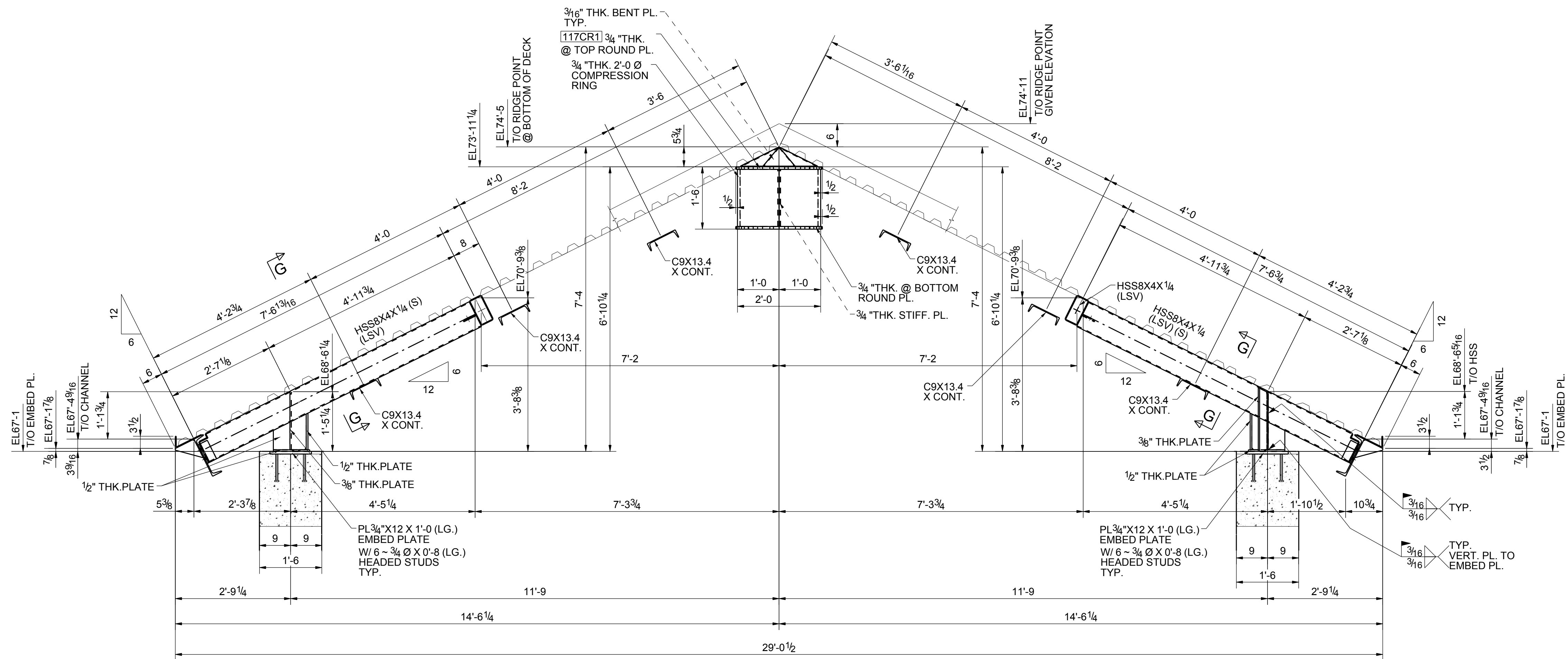
SECTION 7 - 7 1-E103
