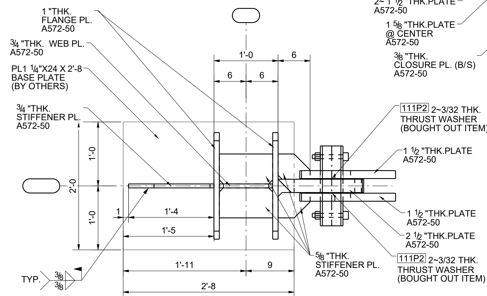
SECTION 57B - 57B
