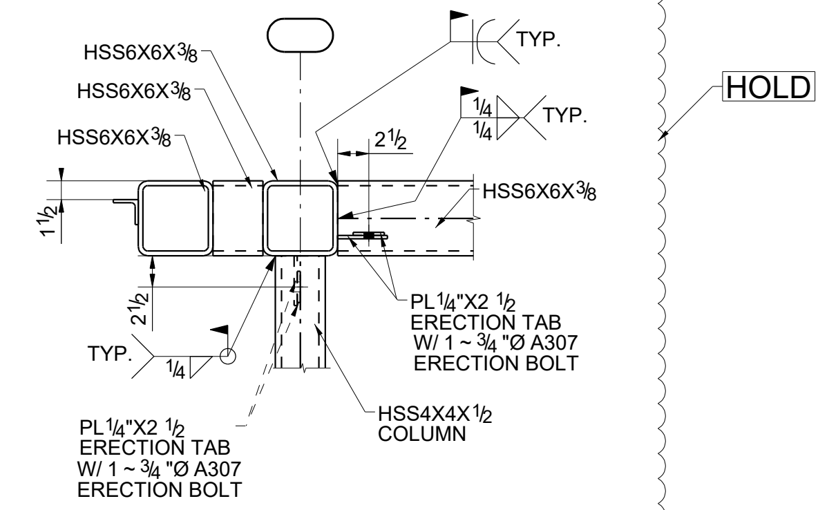
SECTION 17 - 17 E102
