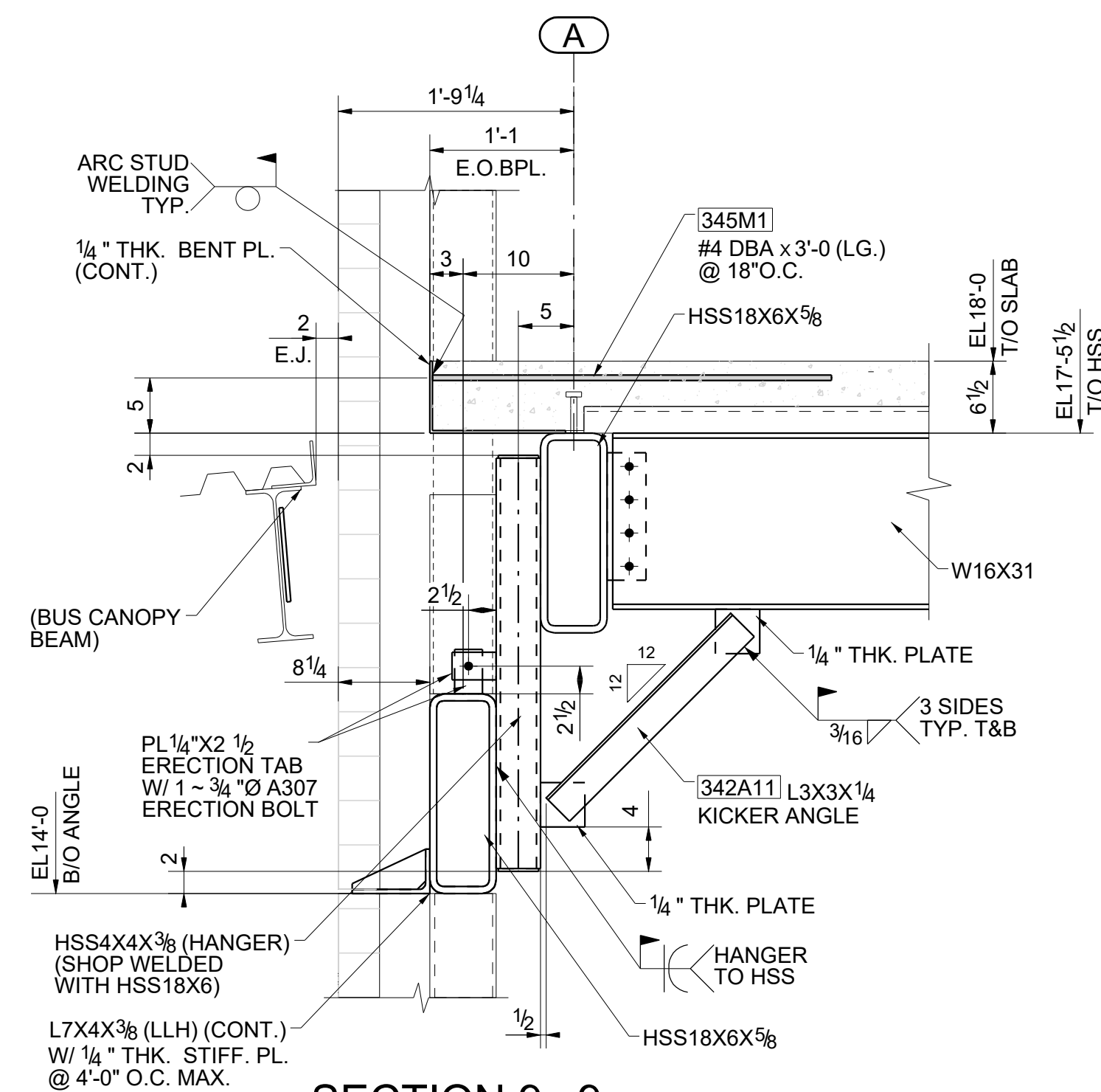
SECTION 9 - 9 E102 (REFER:SECTION 15/S5.006)
