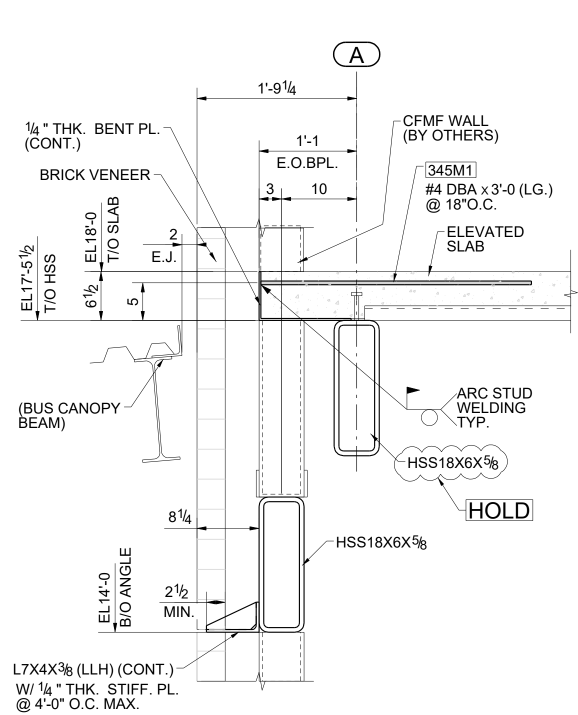
SECTION 8 - 8 E102 (REFER:SECTION 11/S5.006)
