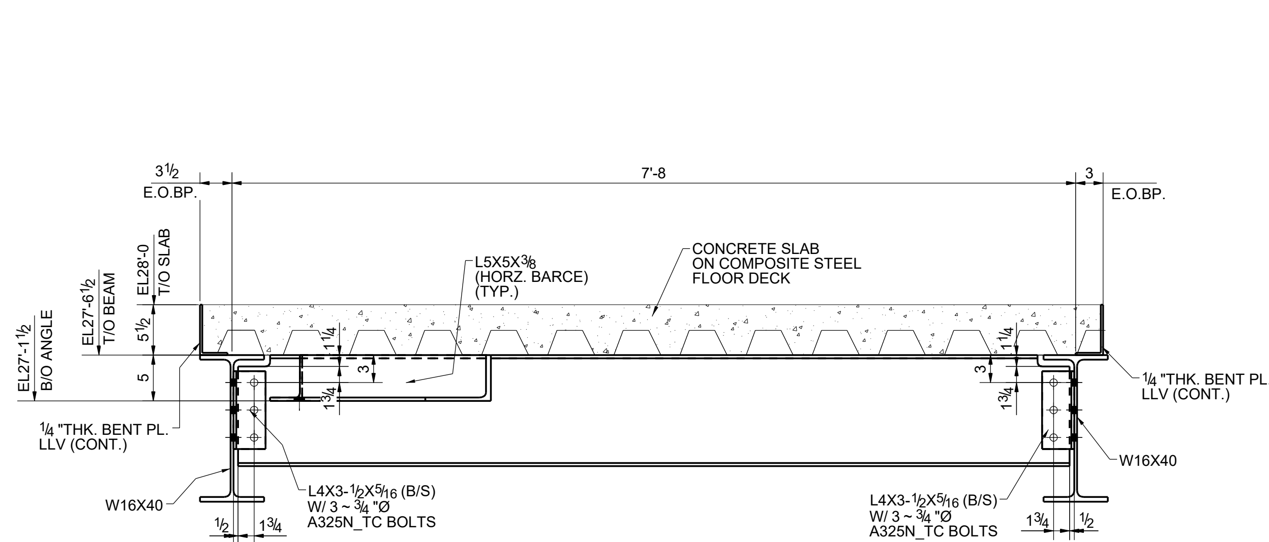
SECTION 84 - 84 E110 (REFER : SECTION 3/S-607)
