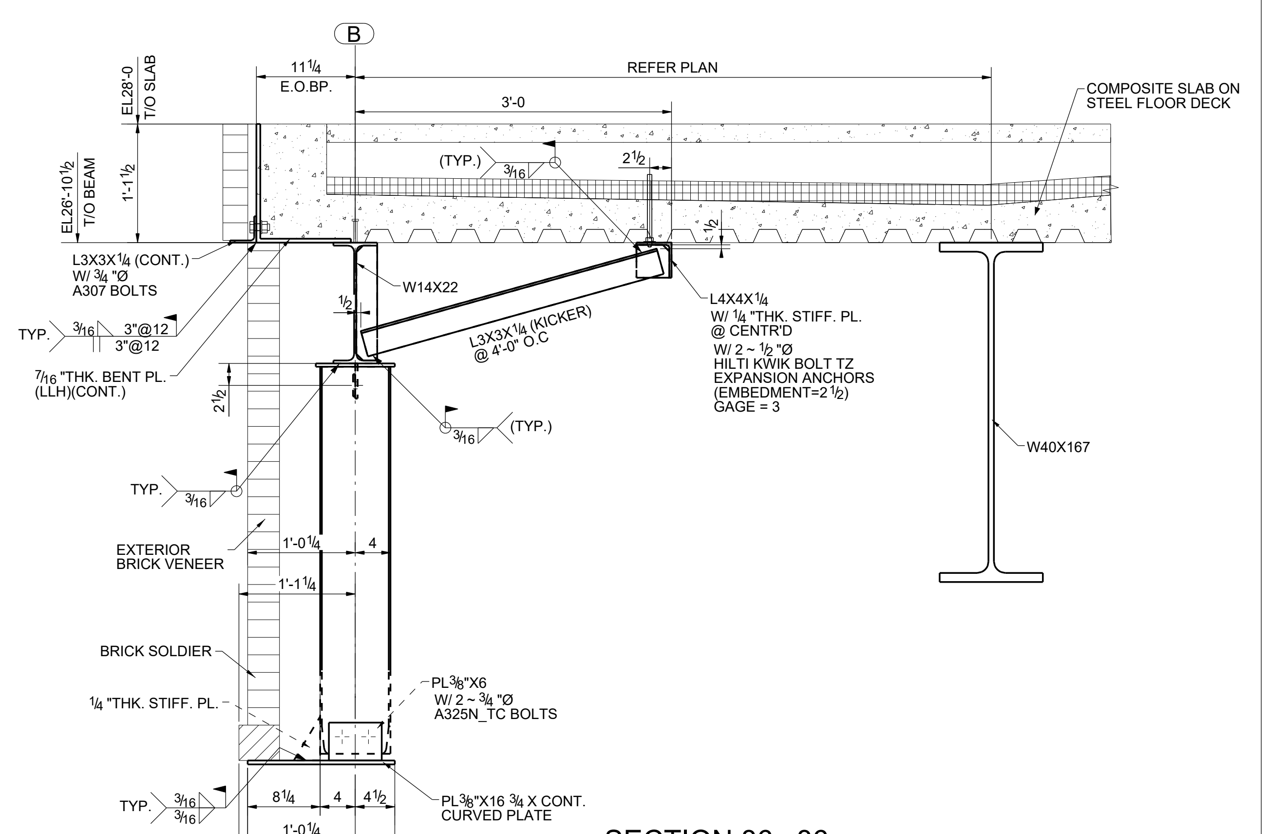
SECTION 86 - 86 E111 (REFER : SECTION 8/S-607)
