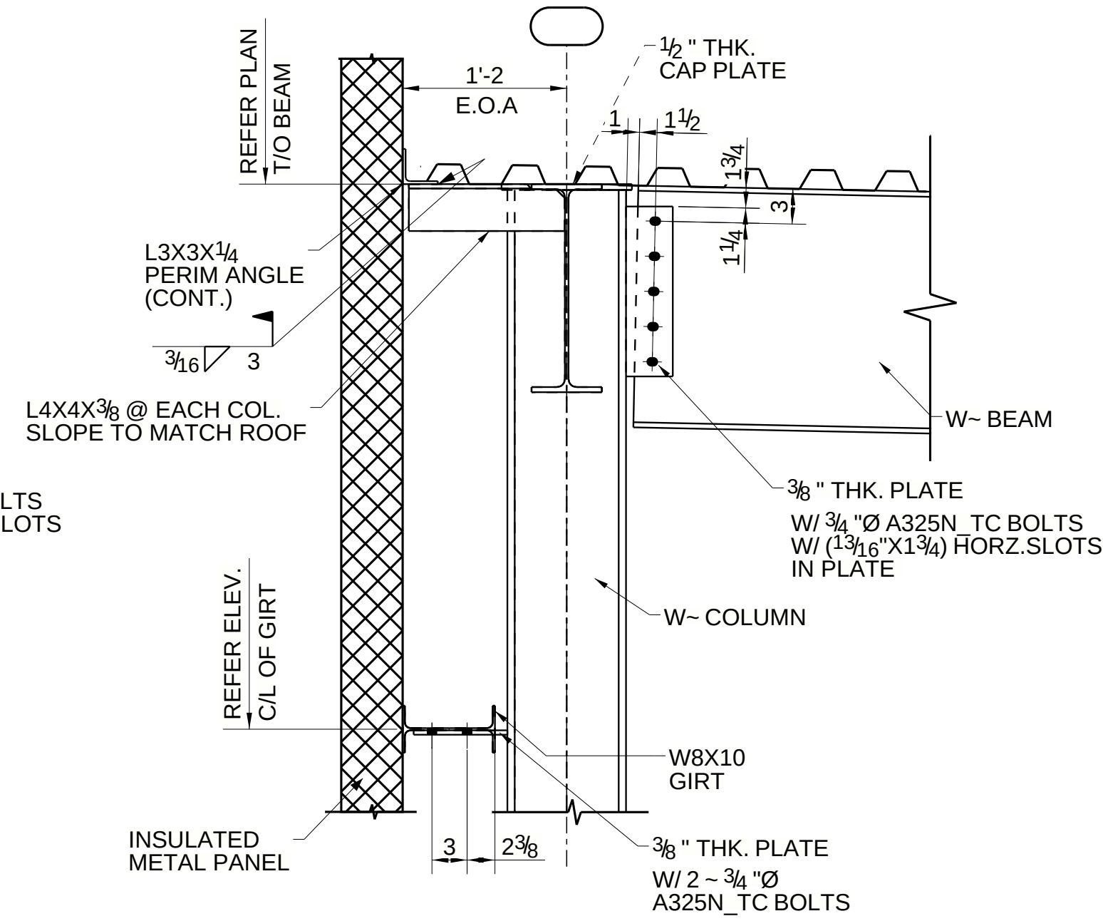
SECTION 28 - 28 E102
