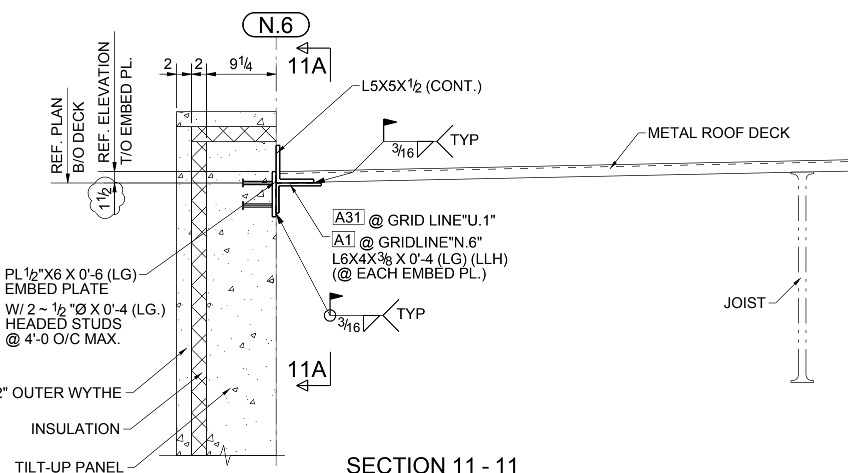
SECTION 11 - 11 E102 & E105
