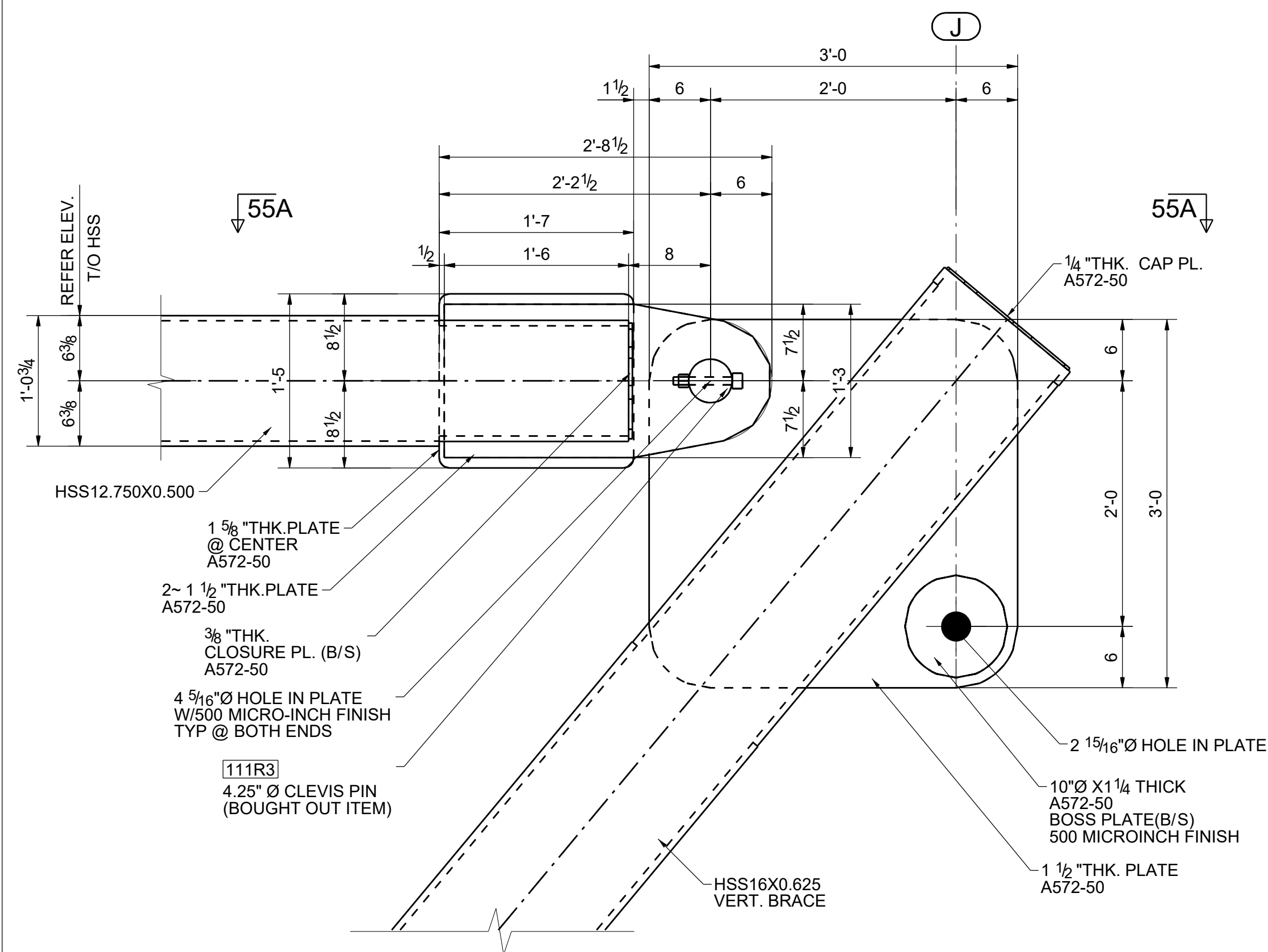
DETAIL 55 E117
