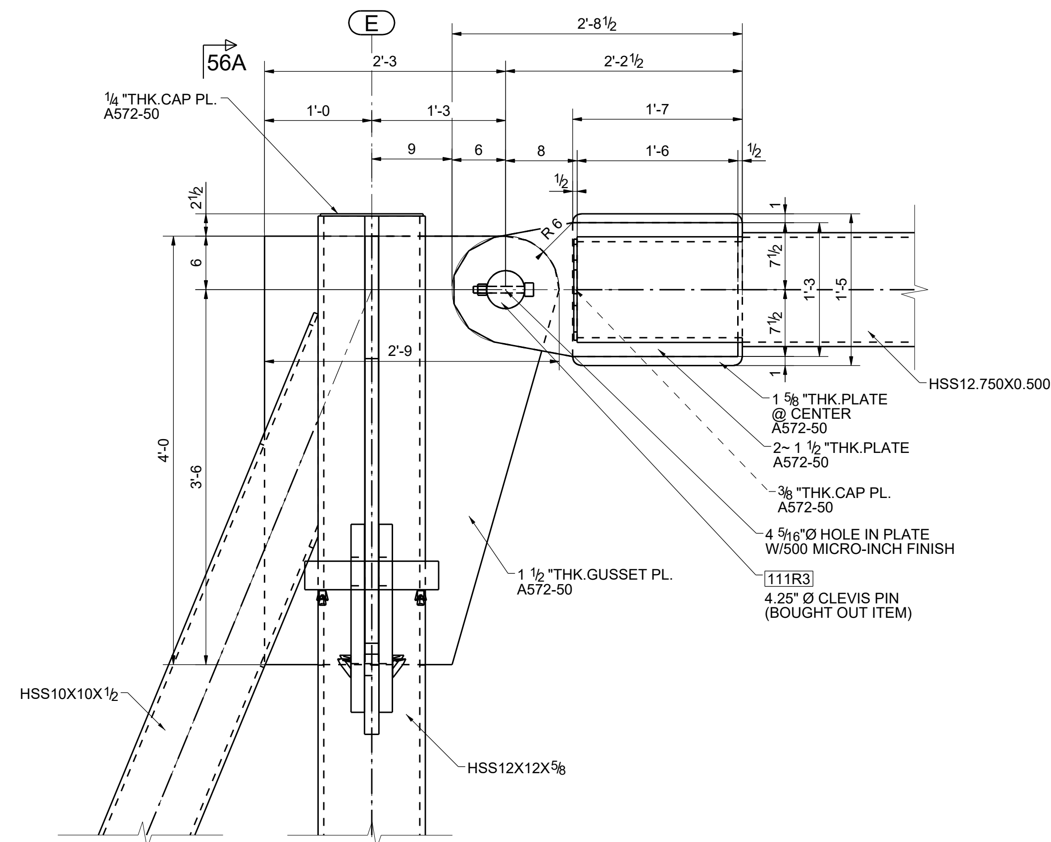
DETAIL 56 - 56 E117
