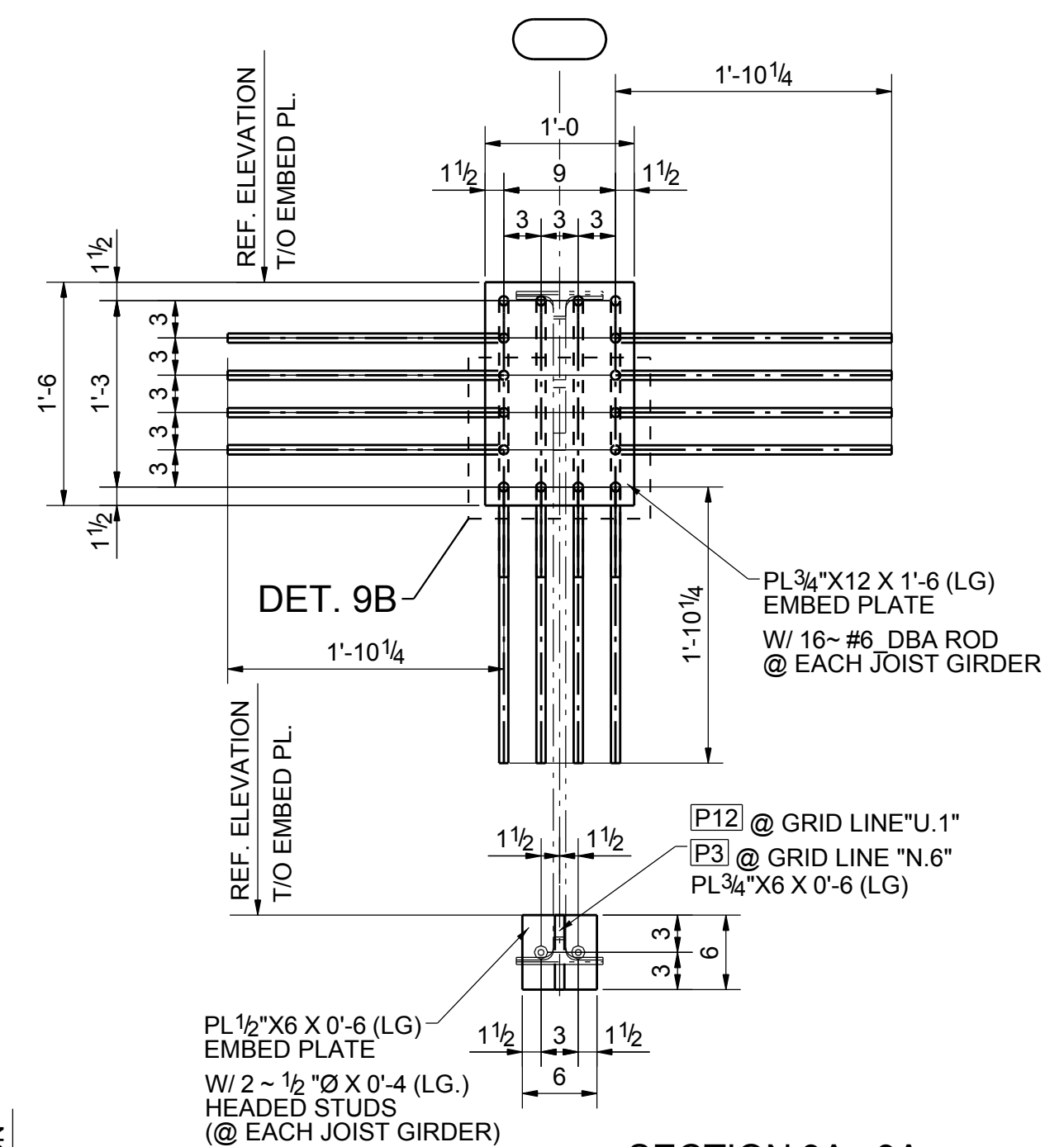
SECTION 9A - 9A
