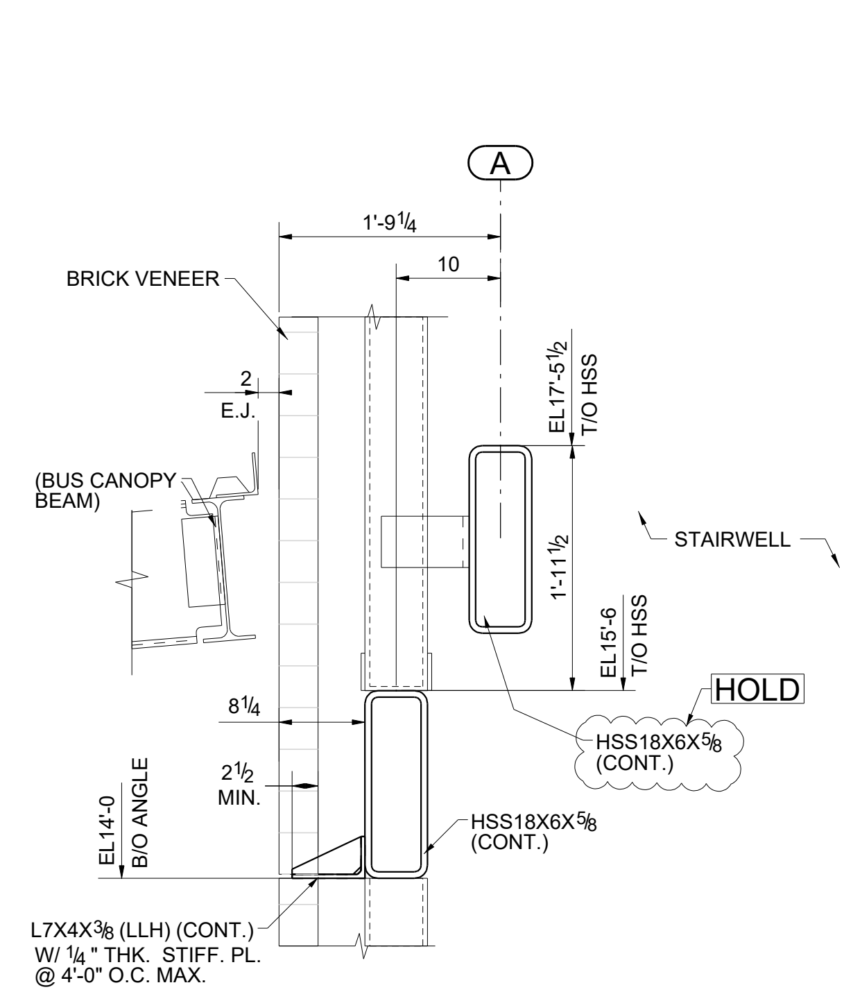
SECTION 7 - 7 E102 (REFER:SECTION 1/S5.006)
