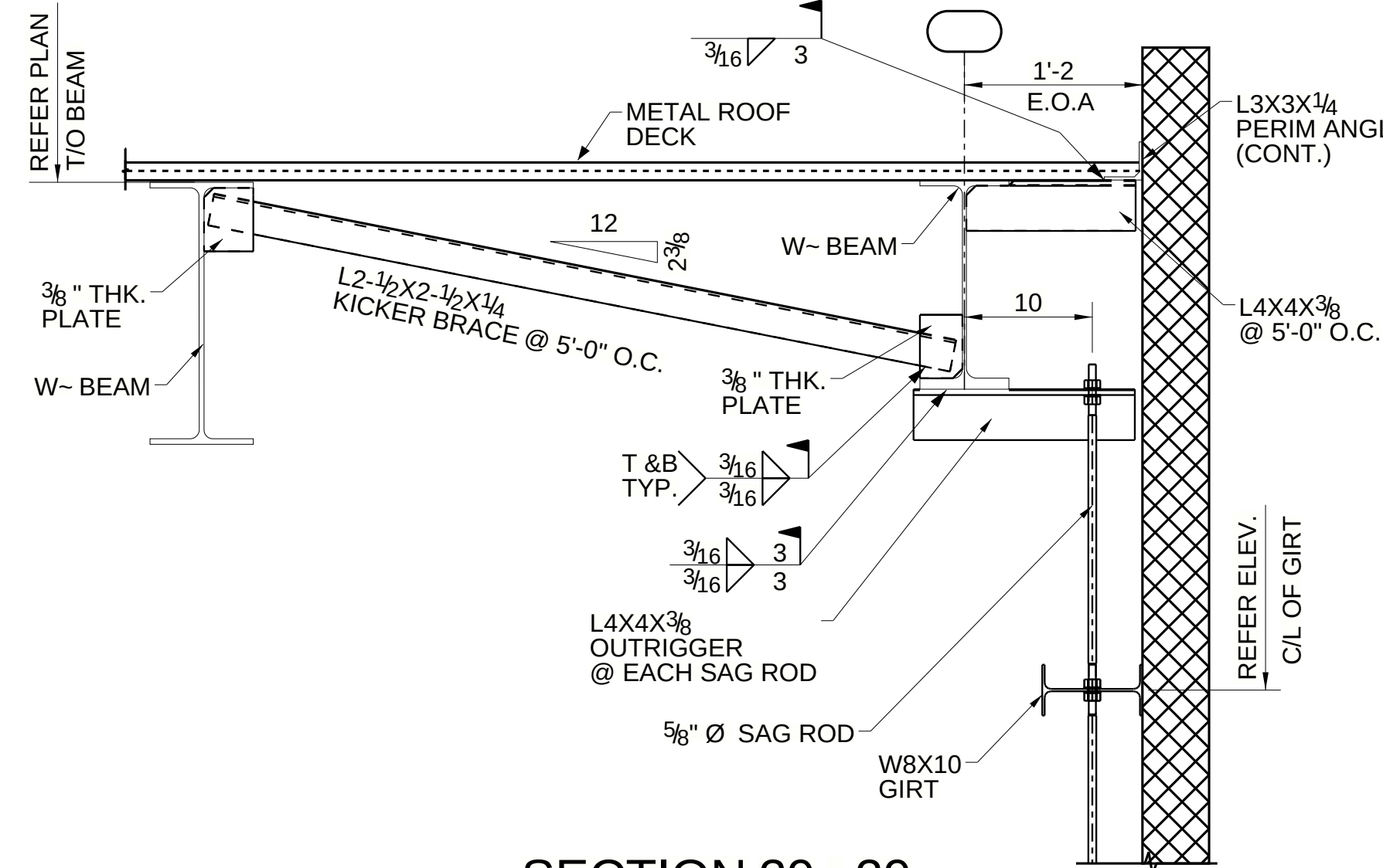
SECTION 29 - 29 E102
