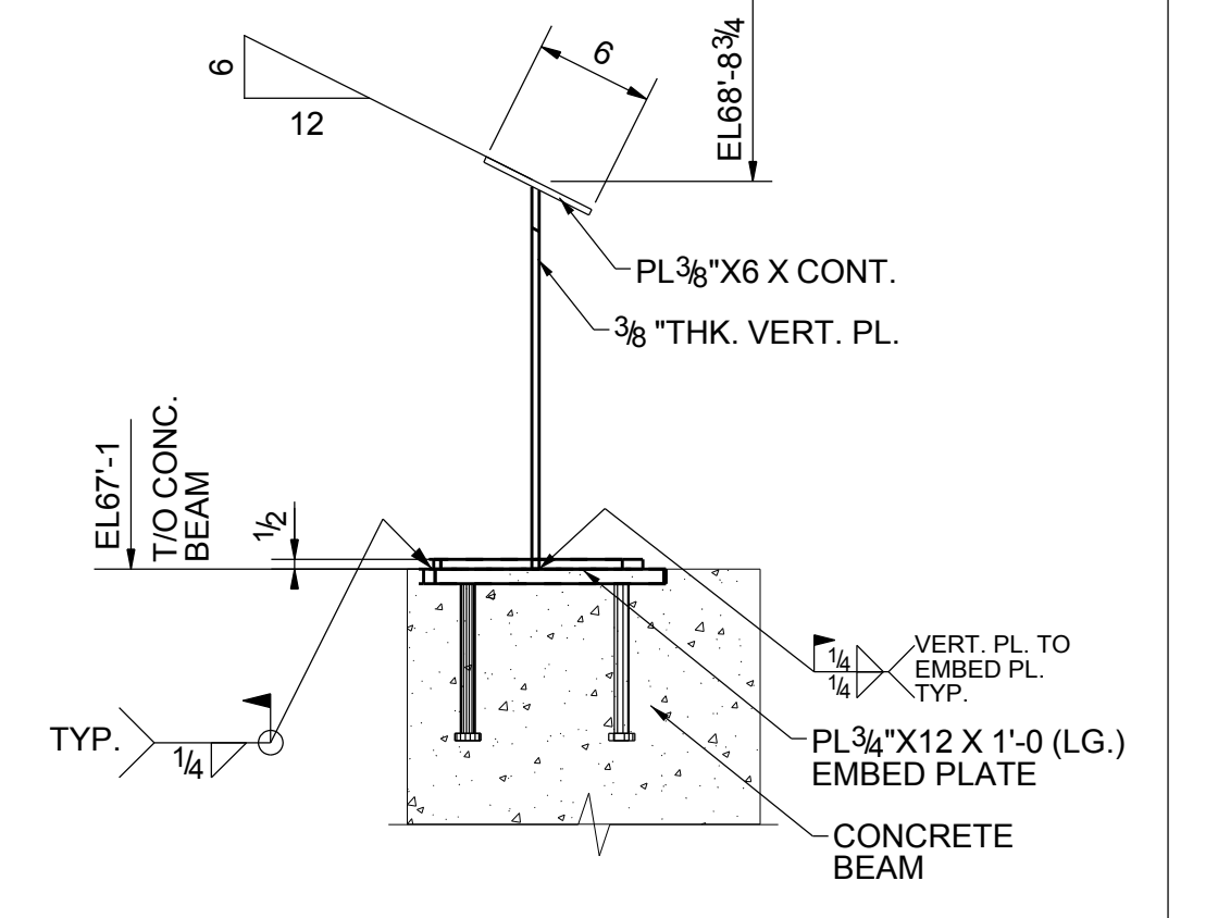
SECTION 10 - 10 1-E103
