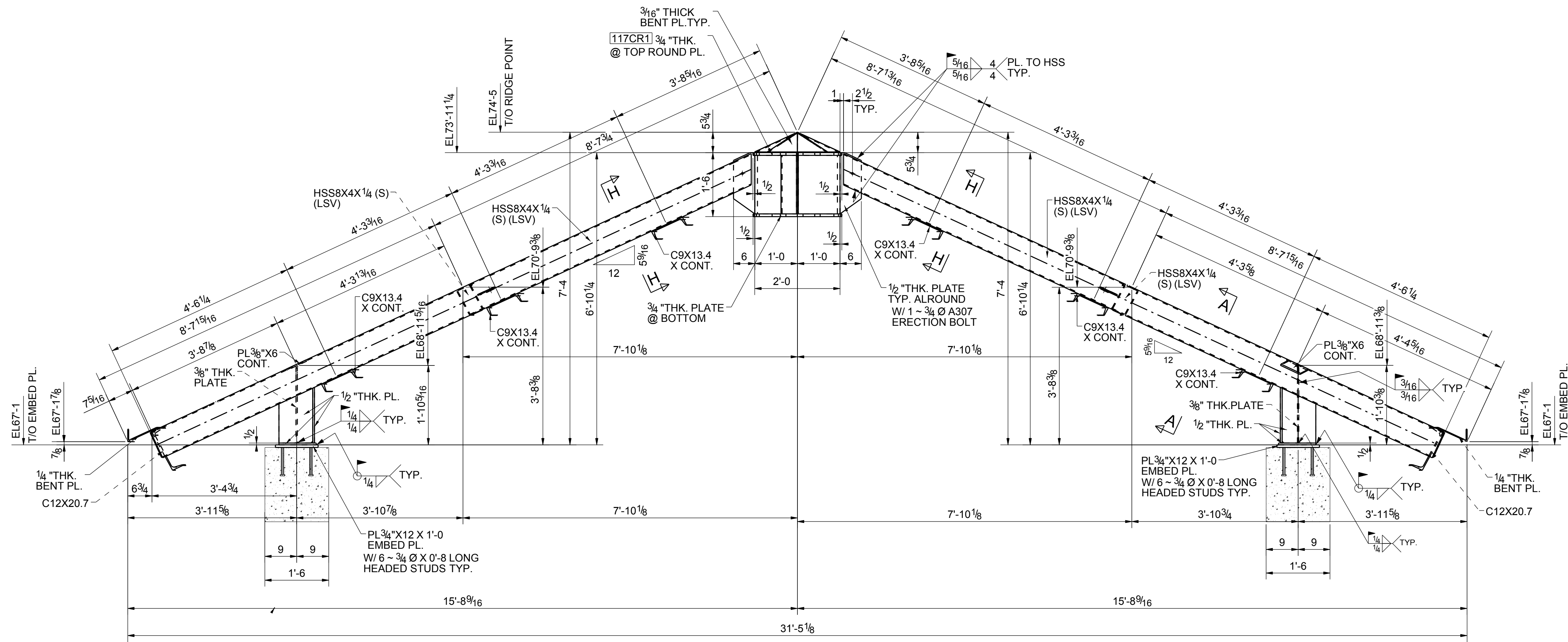
SECTION 8 - 8 1-E103
