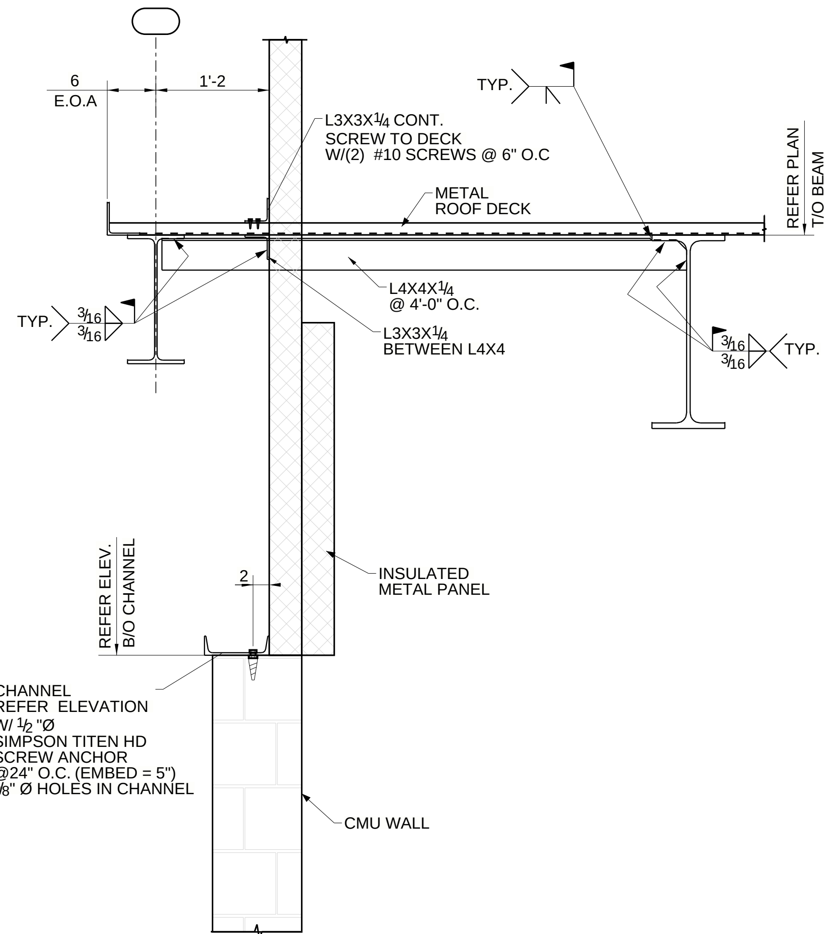
SECTION 31 - 31 E104
