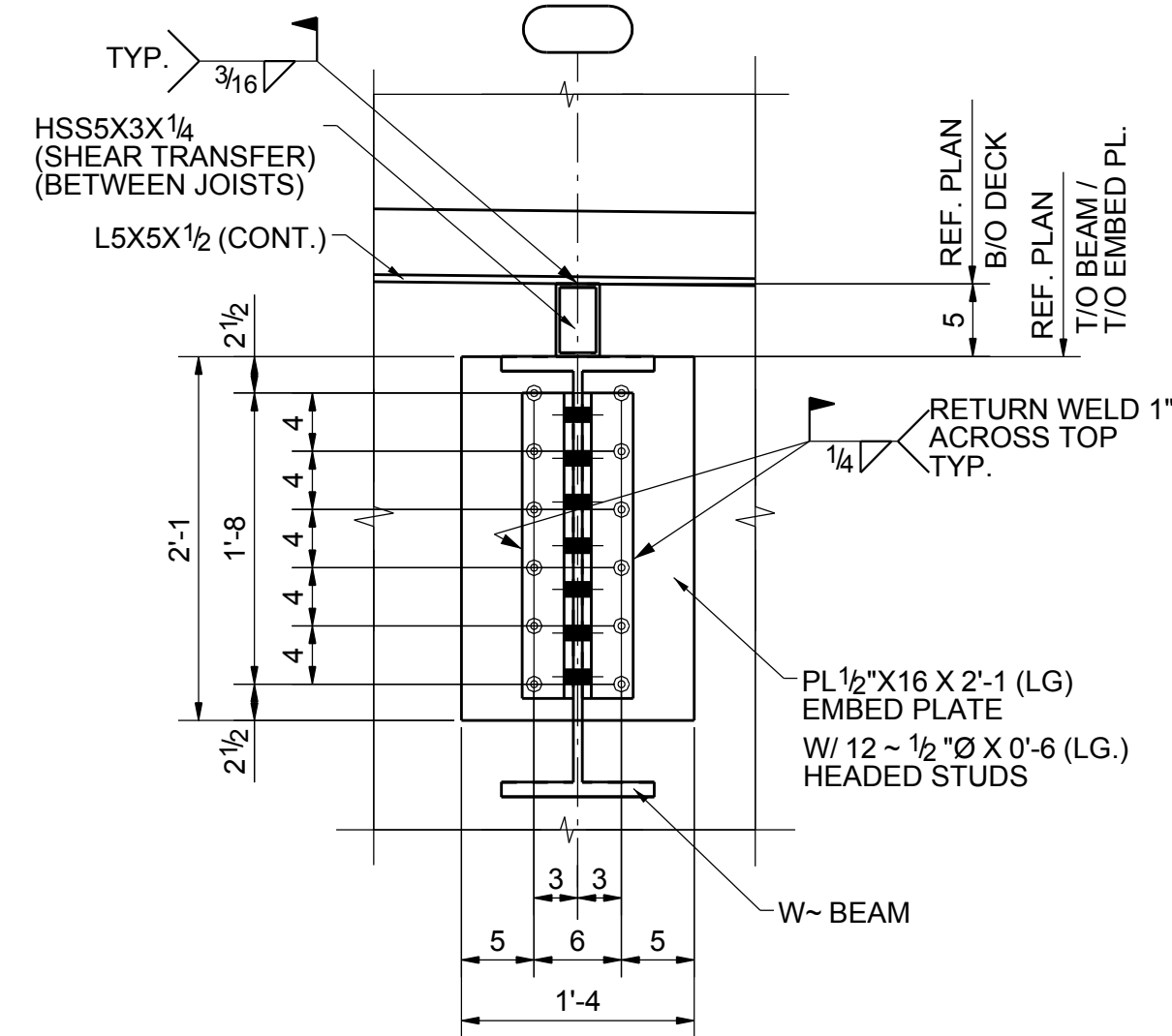
SECTION 8A - 8A
