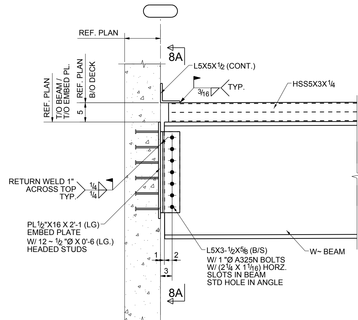
SECTION 8 - 8 E102 & E105
