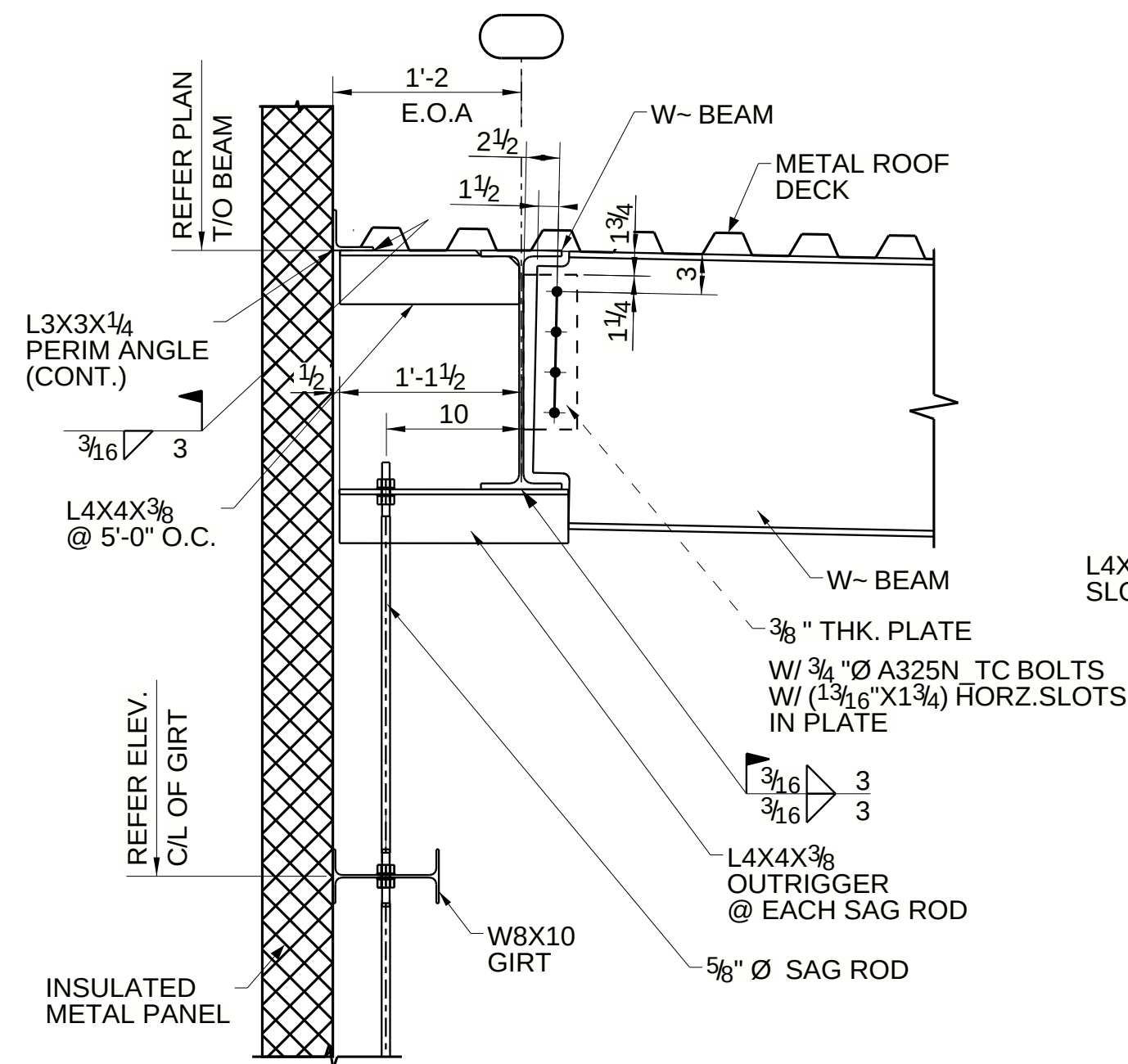
SECTION 27 - 27 E102
