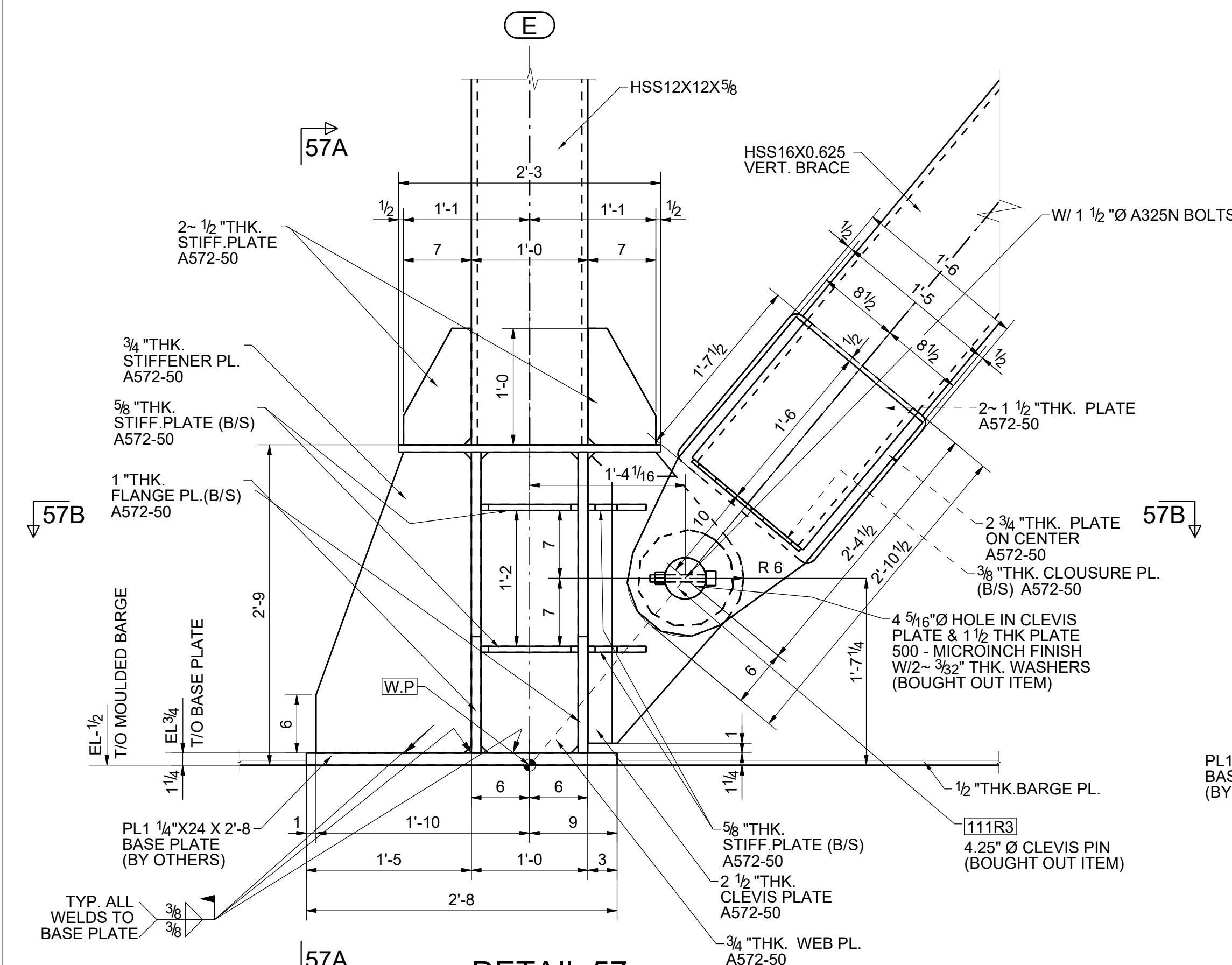
DETAIL 57 E117
