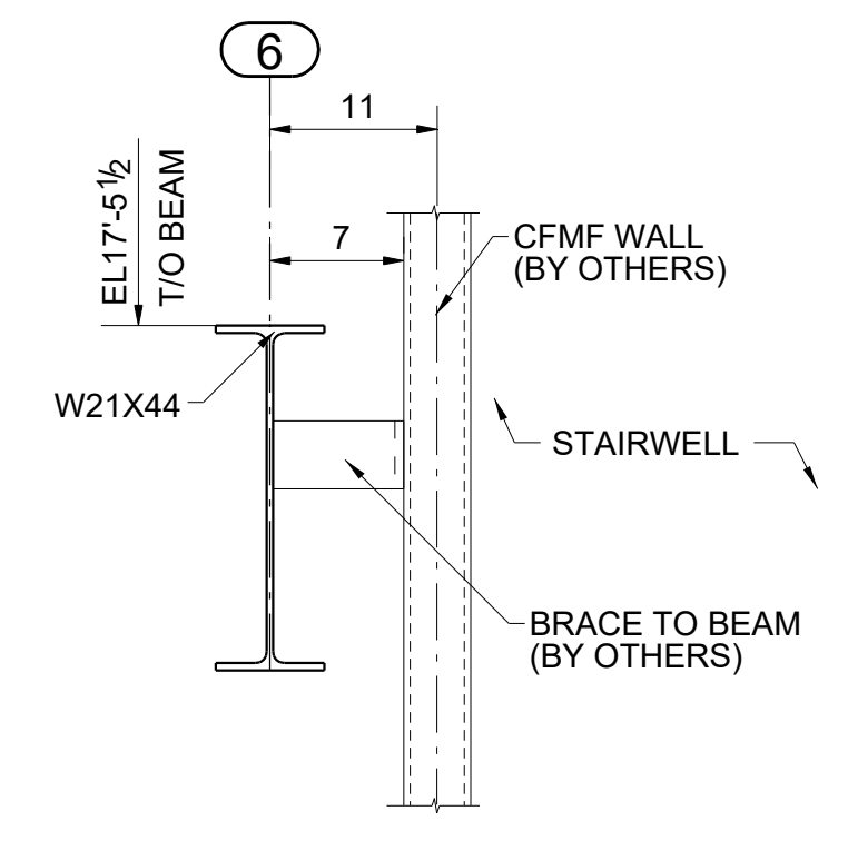
SECTION 15 - 15 E102 (REFER:SECTION 7/S5.007)
