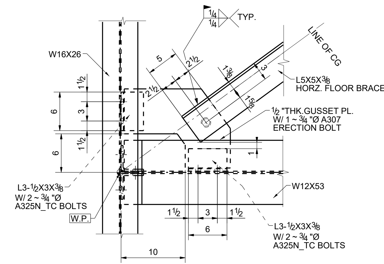
DETAIL 85 E104
